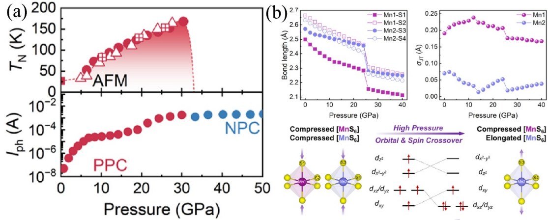
图4 (a) \text{MnSb}_2\text{S}_4 的压强-温度相图, 展示了磁有序温度 ( T_N ) 和光电导电流 ( I_{ph} ) 随压强的变化; (b) \text{MnSb}_2\text{S}_4 中两个不等价的 [\text{MnS}_6] 八面体在压强下的键长变化和八面体畸变演化示意图 [44] 。
